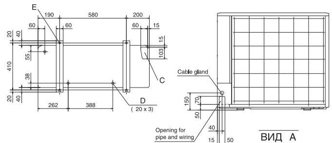
ВИД А
